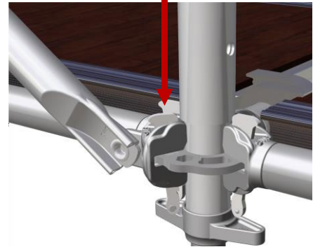
Plateau alu/bois trappe SWS-07-XXXX
