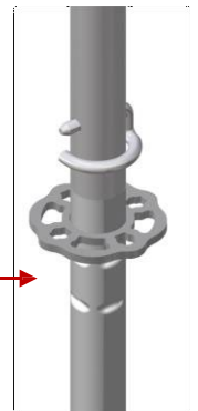
Montant 2 m SWS-02-2001
